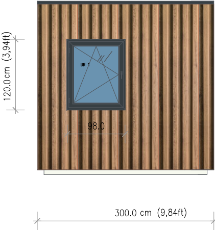
LEFT WALL
